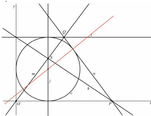
5p 12 Bewijs dat lijn n cirkel c raakt.
